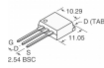
IXTI10N60P IXYS MOSFET N-CH 600V 10A I2-PAK
