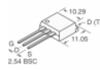
IXTI12N50P IXYS MOSFET N-CH 500V 12A I2-PAK
