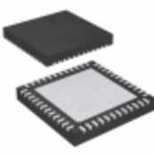
MC9S08RE16FDER NXP USA Inc. IC MCU 8BIT 16KB FLASH 48QFN
