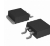
IRF5305SPBF Infineon Technologies MOSFET P-CH 55V 31A D2PAK
