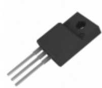
FDPF10N50FT Fairchild/ON Semiconductor MOSFET N-CH 500V 9A TO-220F
