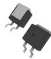
DGSK20-025AS-TUBE IXYS DIODE ARRAY SCHOTTKY 250V TO263
