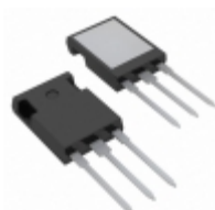
IXFR24N80P IXYS MOSFET N-CH 800V 13A ISOPLUS247
