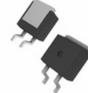
DGS10-018AS IXYS DIODE SCHOTTKY 180V 15A TO263AB
