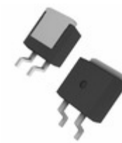
DGS10-018AS-TUBE IXYS DIODE SCHOTTKY 180V 15A TO263AB
