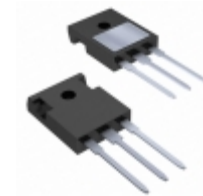
IXTR120P20T IXYS MOSFET P-CH 200V 90A ISOPLUS247
