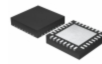
CY8C24423A4-24LTXI Cypress Semiconductor Corp IC MCU 8BIT 4KB FLASH 32QFN
