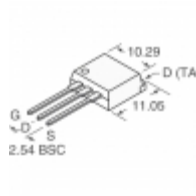
IXTI12N50P IXYS MOSFET N-CH 500V 12A I2-PAK
