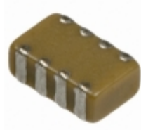
W2A4YA220KAT2A AVX Corporation CAP ARRAY 22PF 16V NP0 0508
