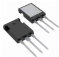
IXFR44N50P IXYS MOSFET N-CH 500V 24A ISOPLUS247
