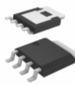
BUK7Y35-55B,115 NXP USA Inc. MOSFET N-CH 55V 28.43A LPAK
