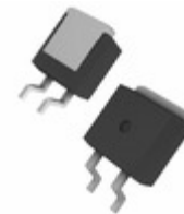
IXTA90N055T2 IXYS MOSFET N-CH 55V 90A TO-263
