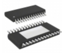
BD63876EFV-E2 Rohm Semiconductor IC MOTOR DRIVER PAR 28HTSSOP
