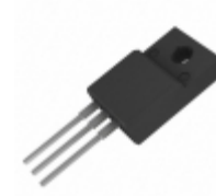
DURF1040CT Littelfuse Inc. DIODE RECTIFIER 5A 400V ITO220AB
