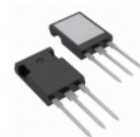
IXFR21N100Q IXYS MOSFET N-CH 1KV 18A ISOPLUS247
