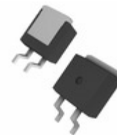
IXTA160N085T IXYS MOSFET N-CH 85V 160A TO-263
