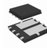
SI7220DN-T1-E3 Vishay Siliconix MOSFET 2N-CH 60V 3.4A 1212-8
