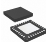
HMC987LP5ETR Analog Devices Inc. IC CLK BUFFER 1:9 8GHZ 32SMT
