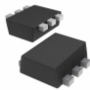
BCM857BV,115 Nexperia USA Inc. TRANS 2PNP 45V 0.1A SOT666
