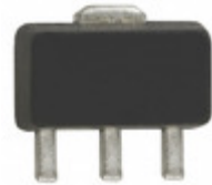
SGA-5389Z RFMD IC AMP HBT SIGE 4500MHZ SOT-89
