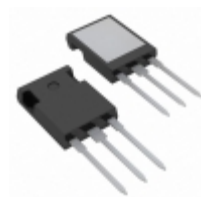
IXGR60N60B2D1 IXYS IGBT 600V 75A 250W ISOPLUS247
