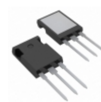
IXTR140P10T IXYS MOSFET P-CH 100V 90A ISOPLUS247
