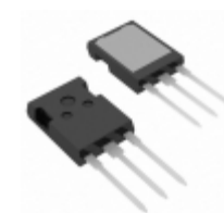
IXFX80N50P IXYS MOSFET N-CH 500V 80A PLUS247
