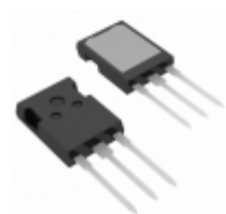
IXFX88N20Q IXYS MOSFET N-CH 200V 88A PLUS247
