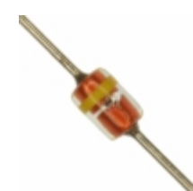
MTZJT-7224C Rohm Semiconductor DIODE ZENER 24V 500MW DO34
