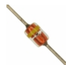
MTZJT-7224B Rohm Semiconductor DIODE ZENER 24V 500MW DO34
