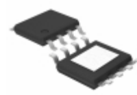
BD60HA3MEFJ-ME2 Rohm Semiconductor IC REG LDO 6V 0.3A 8HTSOP
