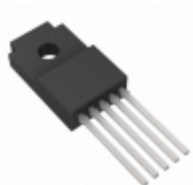
BAJ0CC0WT-F Rohm Semiconductor IC REG LDO 10V 1A TO220FP-5
