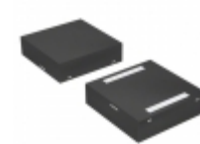
P0900Q22CLRP Hamlin / Littelfuse SIDACTOR BI 75V 400A 2QFN
