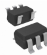
LP2985A-28DBVT N/A IC REG LDO 2.8V 0.15A SOT23-5
