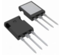
IXFR10N100Q IXYS MOSFET N-CH 1000V 9A ISOPLUS247
