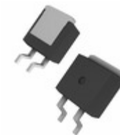
IXTA110N055P IXYS MOSFET N-CH 55V 110A TO-263
