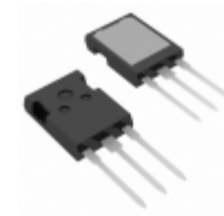
IXTX32P60P IXYS MOSFET P-CH 600V 32A PLUS247
