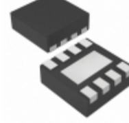
TLV1117-18CDRJR N/A IC REG LDO 1.8V 0.8A 8SON
