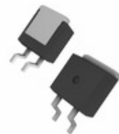
IXTA44P15TTRL IXYS MOSFET P-CH 150V 44A TO-263
