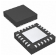
PCA9671BQ,118 NXP USA Inc. IC I/O EXPANDER I2C 16B 24DHVQFN
