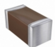
1206GC101KAZ1A AVX Corporation CAP CER 100PF 2KV X7R 1206
