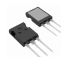
IXTX22N100L IXYS MOSFET N-CH 1000V 22A PLUS247
