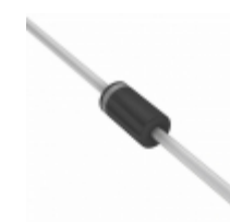
BZW04-23HR1G TSC (Taiwan Semiconductor) TVS DIODE 23.1V 37.5V DO204AL
