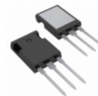
IXFR64N60Q3 IXYS MOSFET N-CH 600V 42A ISOPLUS247
