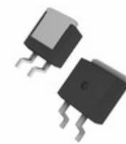
DSS16-01AS IXYS DIODE SCHOTTKY 100V 16A TO263AB
