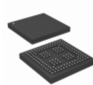
ADSP-21262SKBC-200 Analog Devices Inc. IC DSP 32BIT 200MHZ 136CSBGA
