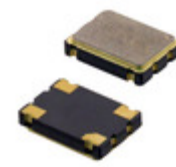
ASV-50.000MHZ-E-T Abracon LLC OSC XO 50.000MHZ HCMOS SMD
