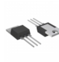
Q2008LH4 Littelfuse Inc. TRIAC ALTERNISTOR 200V 8A TO220
