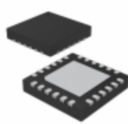
ATSAML10D14A-MUT Micrel / Microchip Technology IC MCU 32BIT 16KB FLASH 24VQFN
