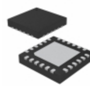
ATSAML10D15A-MUT Micrel / Microchip Technology IC MCU 32BIT 32KB FLASH 24VQFN
