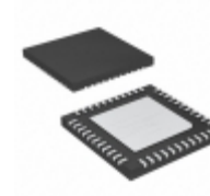
PIC18LF442T-I/ML Microchip Technology IC MCU 8BIT 16KB FLASH 44QFN
