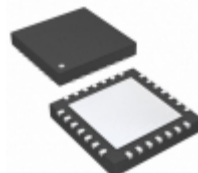
PIC18LF24J11T-I/ML Microchip Technology IC MCU 8BIT 16KB FLASH 28QFN
