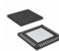
ATXMEGA16D4-MHA2 Microchip Technology IC MCU 8BIT 16KB FLASH 44VQFN
