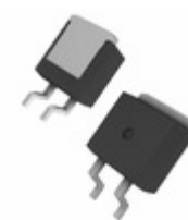
DSEI36-06AS-TUB IXYS DIODE GEN PURP 600V 37A TO263AB
