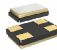
FA-238 27.0000MA-C3 EPSON CRYSTAL 27.00 MHZ 18.0PF SMD
